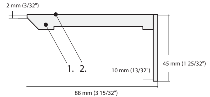
L-CASING
