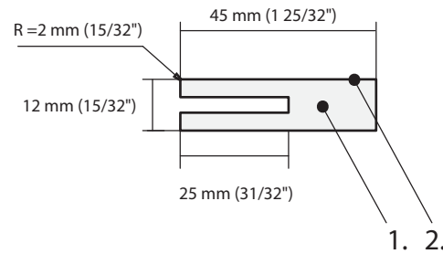
SPLIT JAMB
